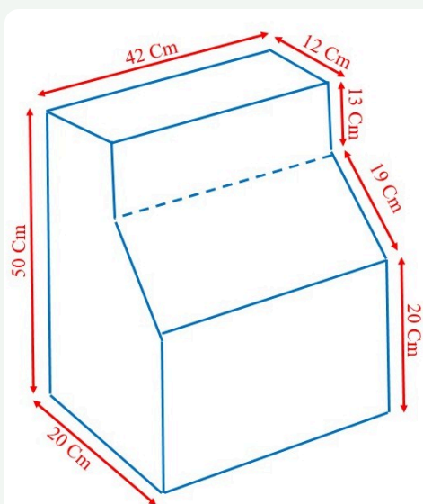
نقشه ابعادی – تمام اندازه‌ها (سانتی‌متر)
