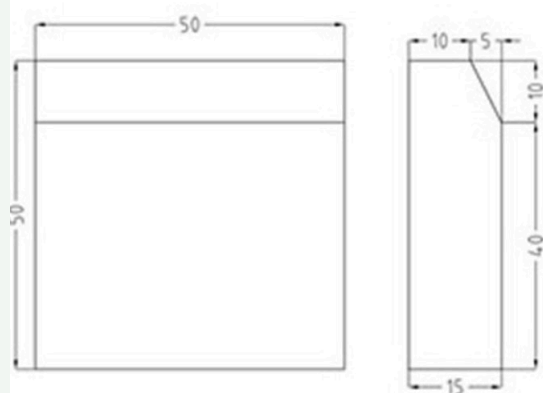
نقشه ابعادی – نمای روبه‌رو و جانبی (سانتی‌متر)
